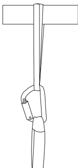
Afb. 1A: Horizontale verankering
